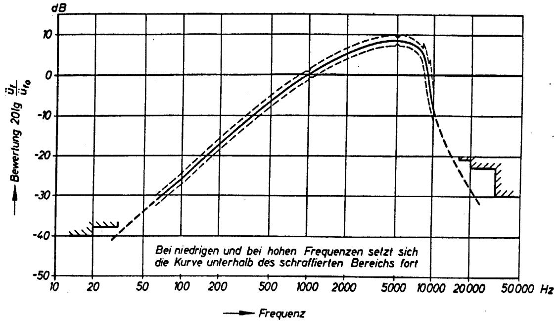
Bewertungsfaktoren des Geräuschspannungsmessers für elektroakustische Breitbandübertragung
